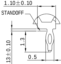
DETAIL PIN2 SCALE 10:1
